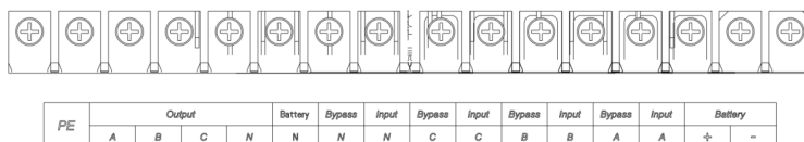
(б) Силовые клеммы ИБП мощностью 10-60 кВА с отсеком для встроенных АКБ
