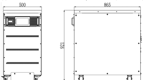
(г) 10; 15; 20; 30 кВА с отсеком для встроенных АКБ (ед. изм.: мм)
