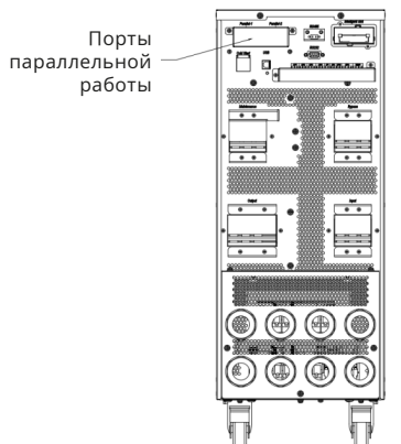
Рисунок 5.4. Расположение коммуникационных портов параллельной работы
