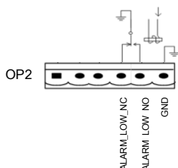
Рисунок 3.14. Схема интерфейса выходного релейного контакта общей тревоги
