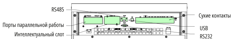
(г) 60 кВА с отсеком для встроенных АКБ
