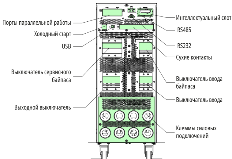
(д) ИБП мощностью 40/60 кВА без отсека для встроенных АКБ, вид сзади
